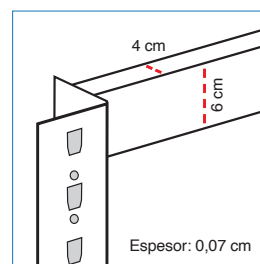
8 Vigas
