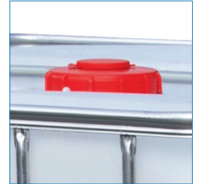
Tapa de llenado DN 150 con tapa rosca con venteo
