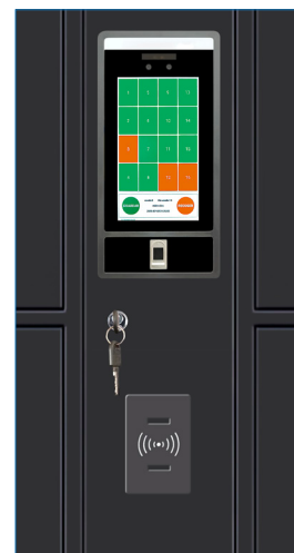
Pantalla LCD Lector de huella Lector Tarjeta RFID
